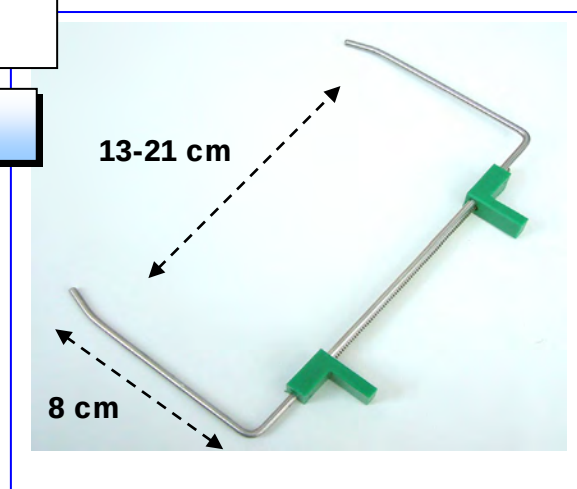
PINZA SPACCHI INOX VENT CLAMP INOX PINCE FENTES INOX
